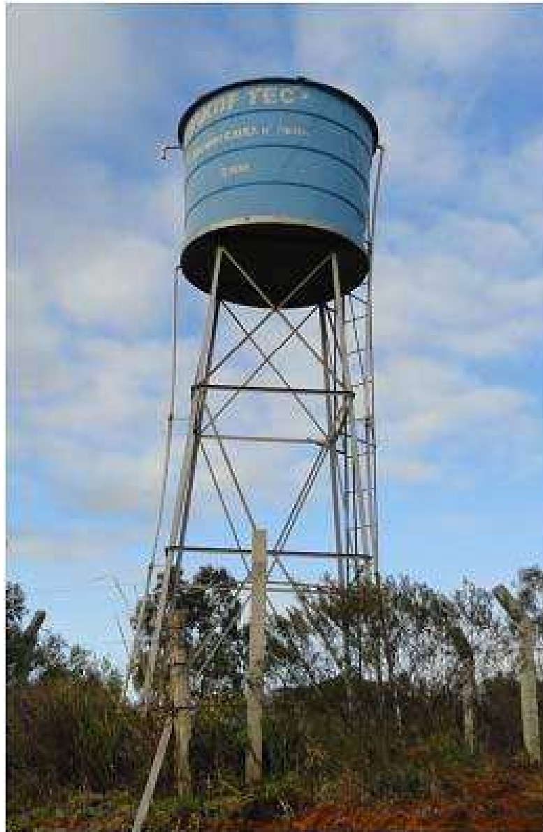
Ilustração 023 – Por último, outra caixa d'água, também de 5.000 litros, é abastecida, indiretamente, pelo MB-3. Serve, também, como amortecimento de energia da água e possui tubulações de entrada e saída com mesmo diâmetro, ambas DN 50.
