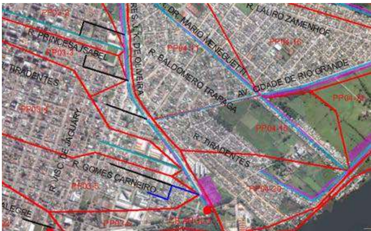
Figura 57: Proposições de Macrodrainagem para o trecho de jusante das sub-bacias PP-03 e PP-04.
